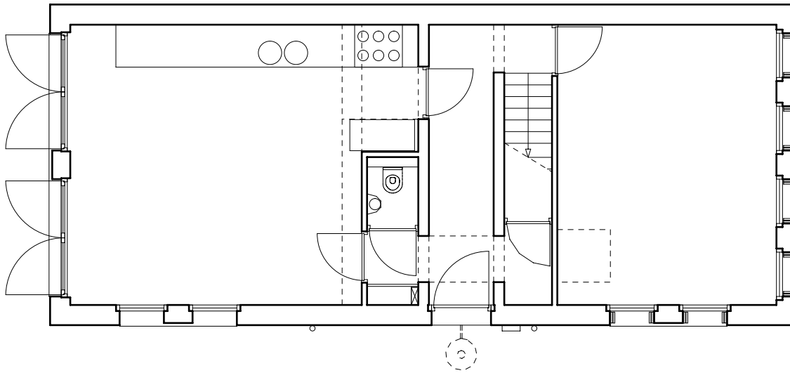
BEGANE GROND
